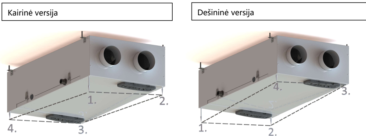
Pav. 3. Horizontalaus montavimo schema
